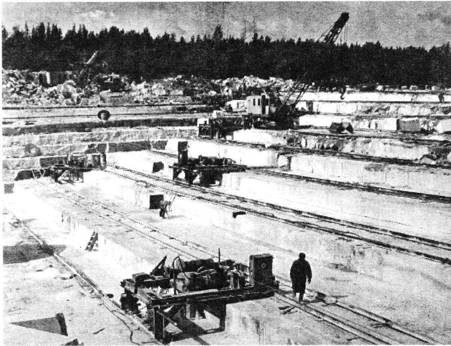
Механизированная добыча мрамора.
